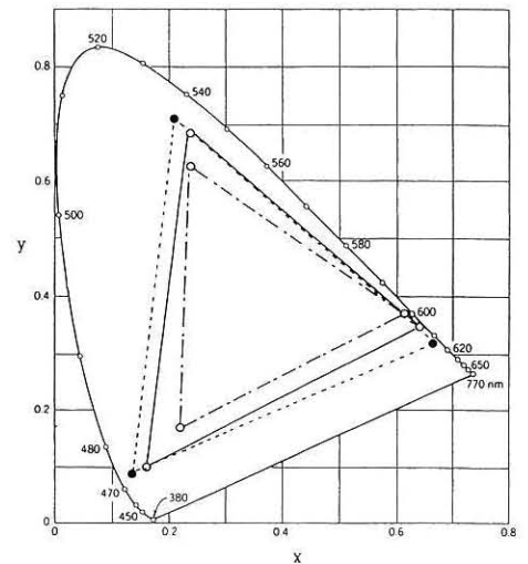
図3:Autochrome Plate(AC-1, AC-2)の微小フィルターに関するCIE色度座標(平均値)および参照としてのNTSCカラーテレビ原色の色度座標
