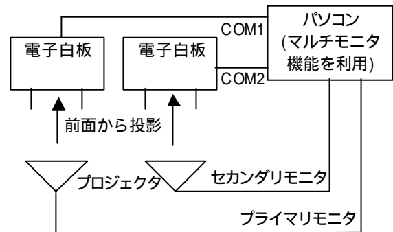
図1 ハードウェア構成(前面投影型電子白板)
