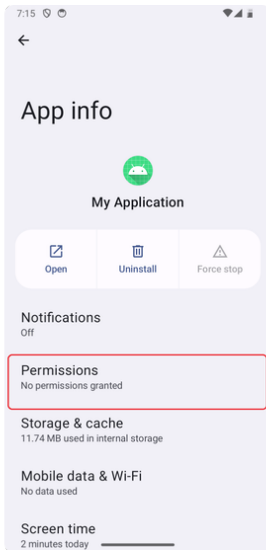
図 4.6.7 READ_MEDIA_IMAGES 権限が付与されていない
