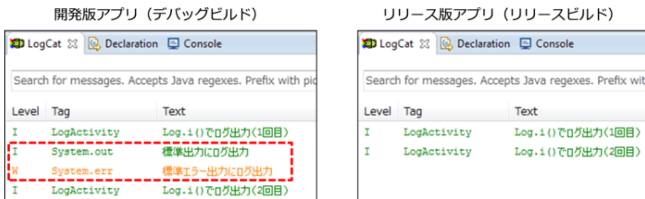
図 4.8.3 System.out/err の開発版アプリとリリース版アプリの LogCat 出力の違い
