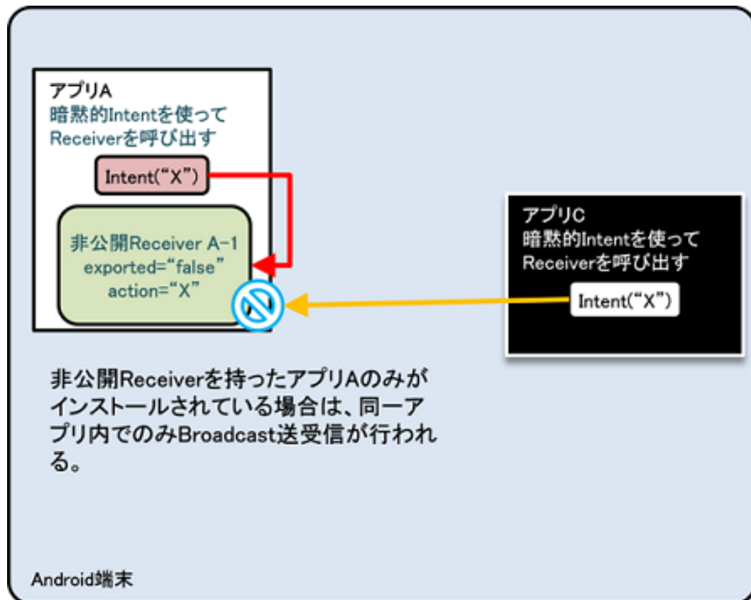
図 4.2.4 正常な動作の例
