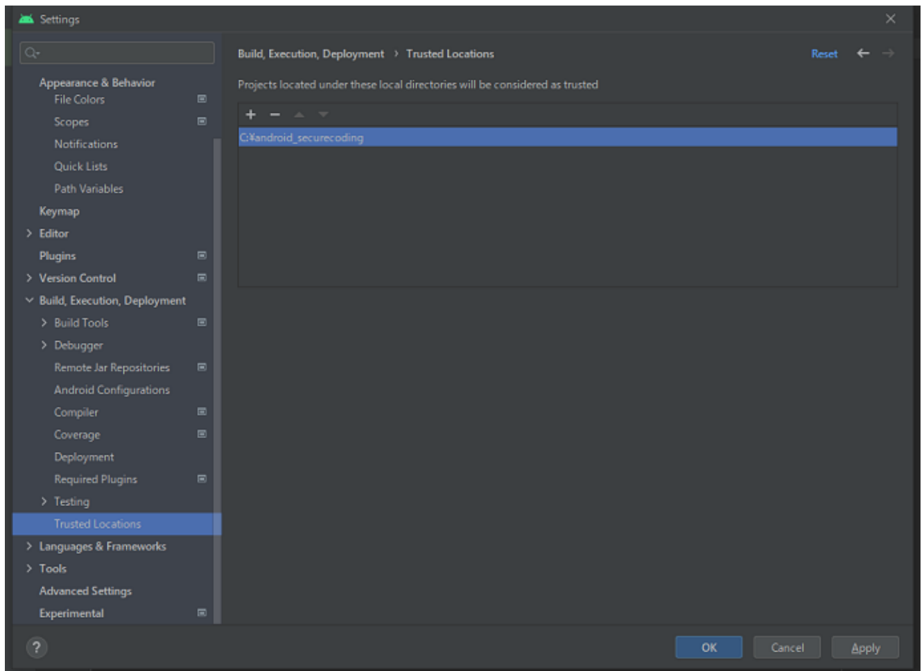
図 2.5.23 C:\android_securecoding を追加
