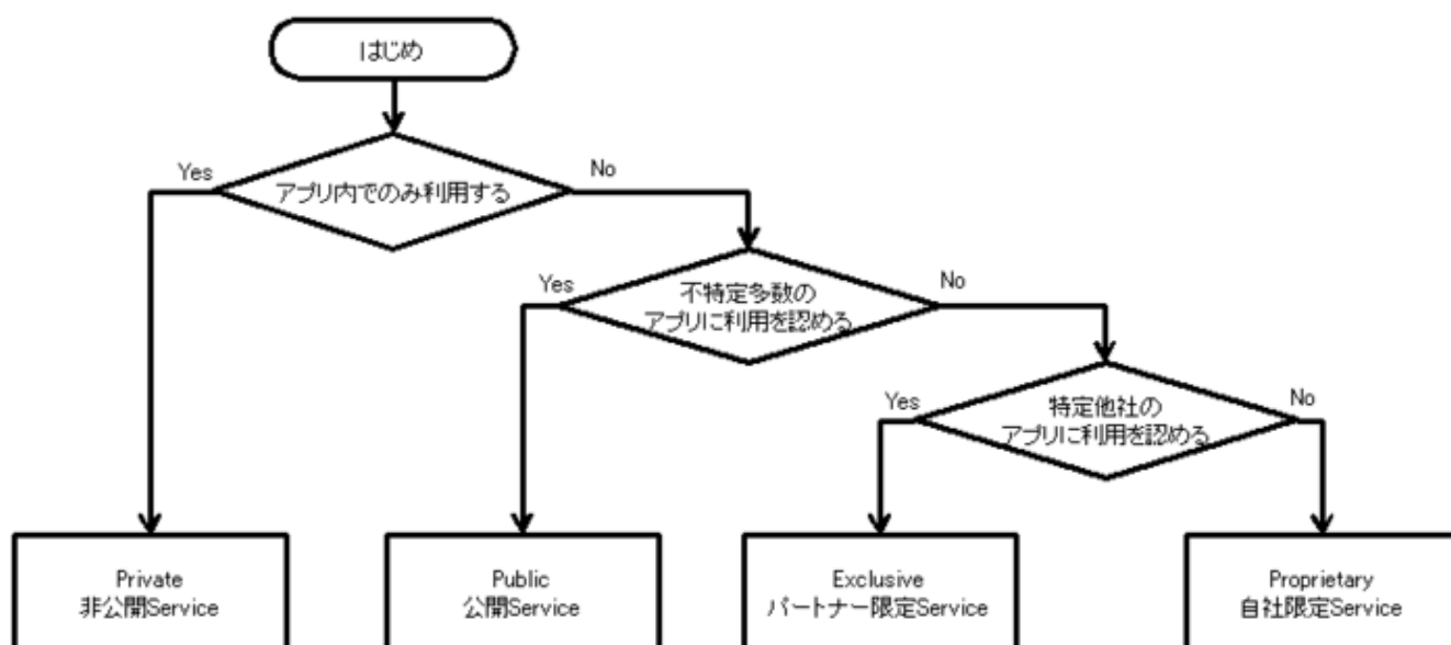
図 4.4.1 Service タイプの選択フロー
