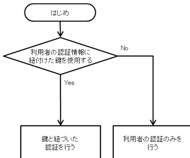
図 5.7.1 生体認証を利用するサンプルコード選択フローチャート
