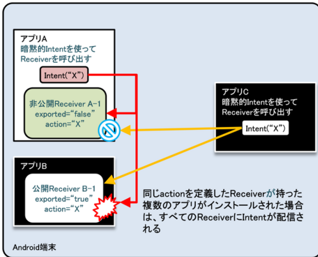
図 4.2.5 意図しない動作の例
