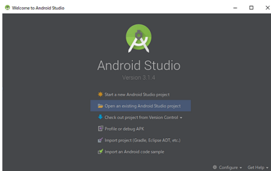
図 2.5.7 Open project
