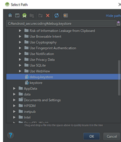
Fig. 2.5.16: Select “debug.keystore”
