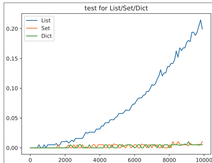
図 76: spdTest02.py の実行結果 横軸はデータの個数，縦軸は実行時間
