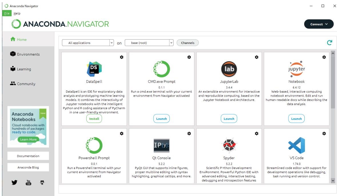
図 49: Anaconda Navigator
