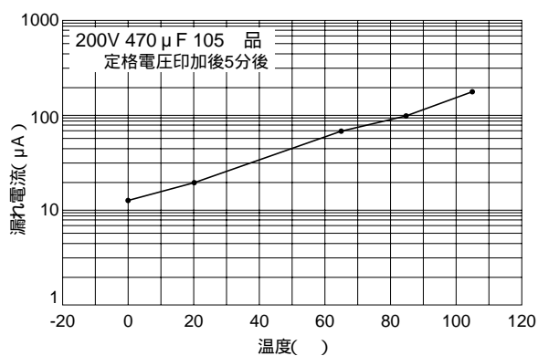
図 1-12 漏れ電流の温度特性
