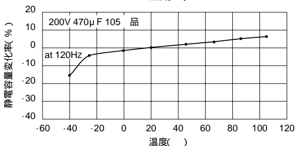
図 1-9 静電容量の温度特性
