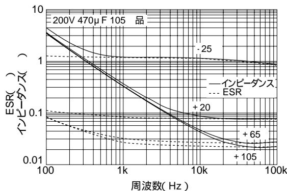
図 1-11 インピーダンス, ESRの周波数特性
