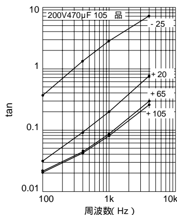
図 1-10 tan の周波数特性
