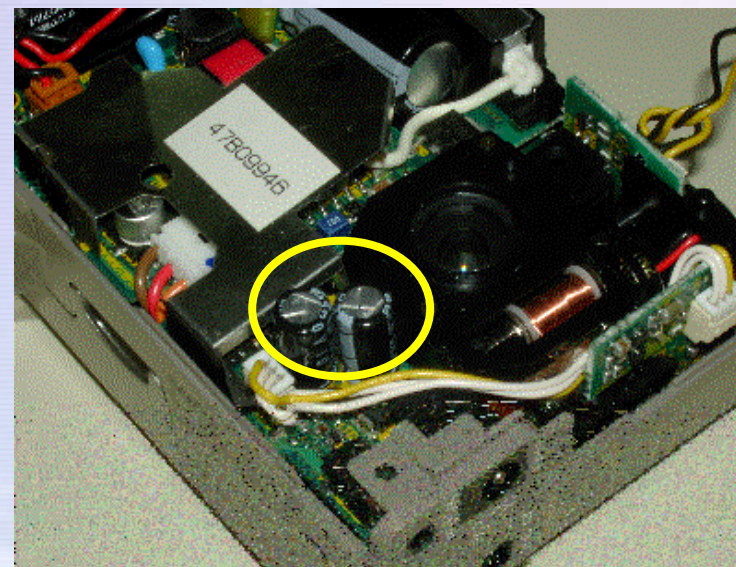
アルミ電解コンデンサ 10V/330uF(2p) Φ 6.3mm × L11.0mm
