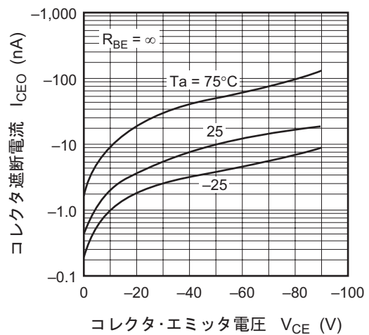
コレクタ遮断電流対 コレクタ・エミッタ電圧特性
