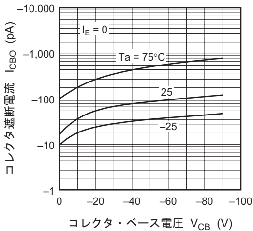
コレクタ遮断電流対 コレクタ・ベース電圧特性
