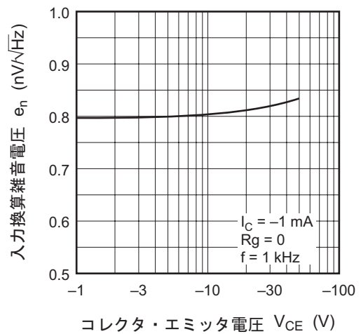
入力換算雑音電圧対 コレクタ・エミッタ電圧特性
