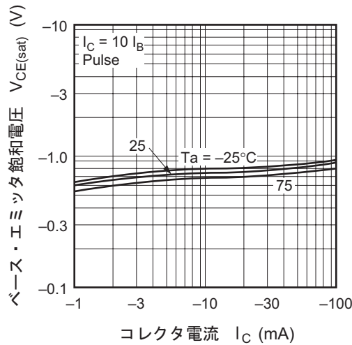
ベース・エミッタ飽和電圧対 コレクタ電流
