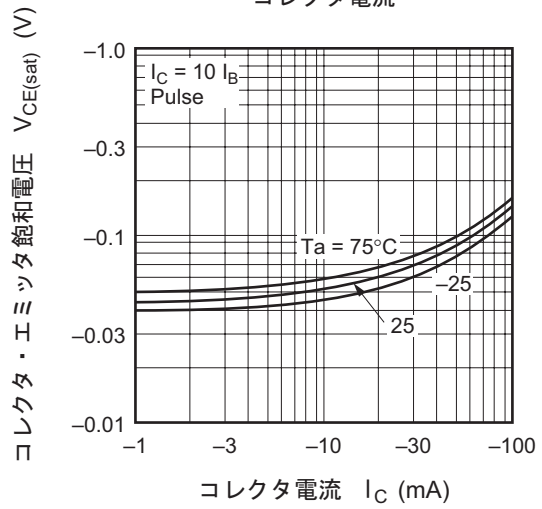
コレクタ・エミッタ飽和電圧対 コレクタ電流
