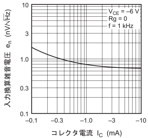
入力換算雑音電圧対コレクタ電流 特性
