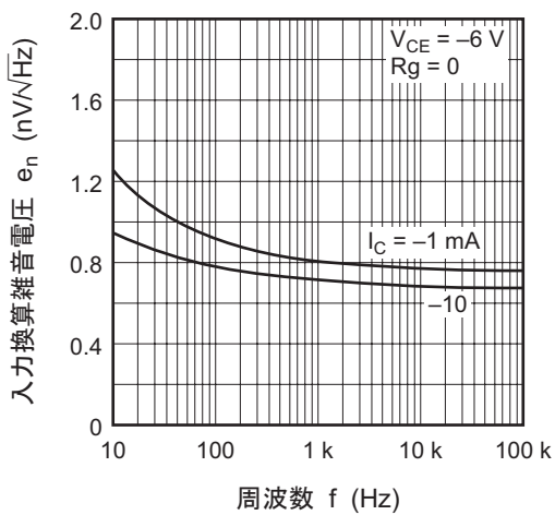
入力換算雑音電圧対周波数特性
