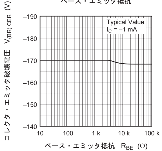
コレクタ・エミッタ破壊電圧対 ベース・エミッタ抵抗
