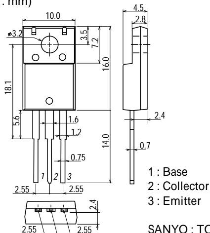
外形図 2041A
