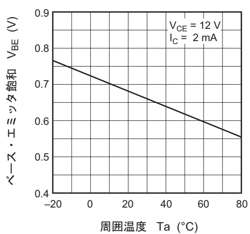
ベース・エミッタ電圧対周囲温度特性
