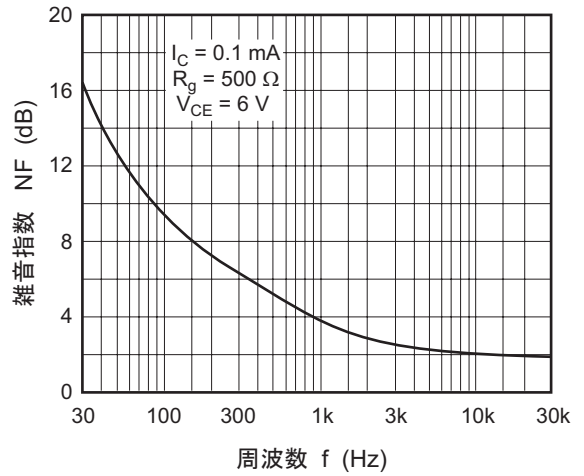
雑音指数対周波数特性
