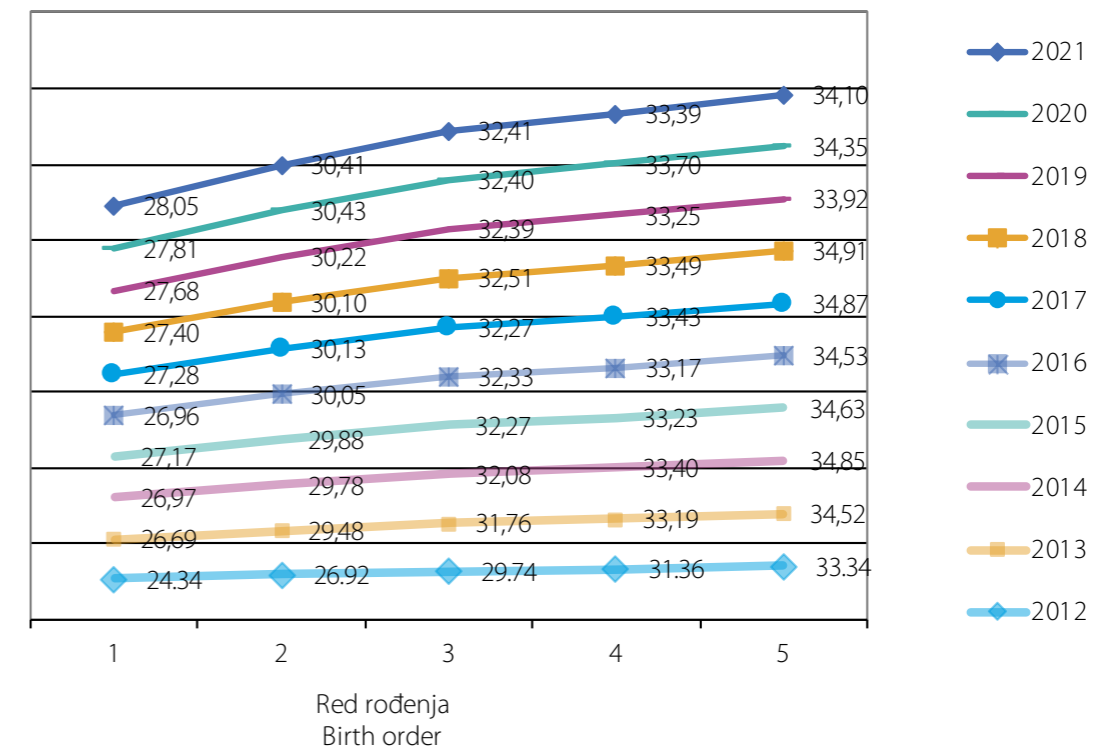
Grafikon 4. Prosječna starost majke prema redu rođenja živorođene djece Graph 4. Average mother's age by birth order of live births
