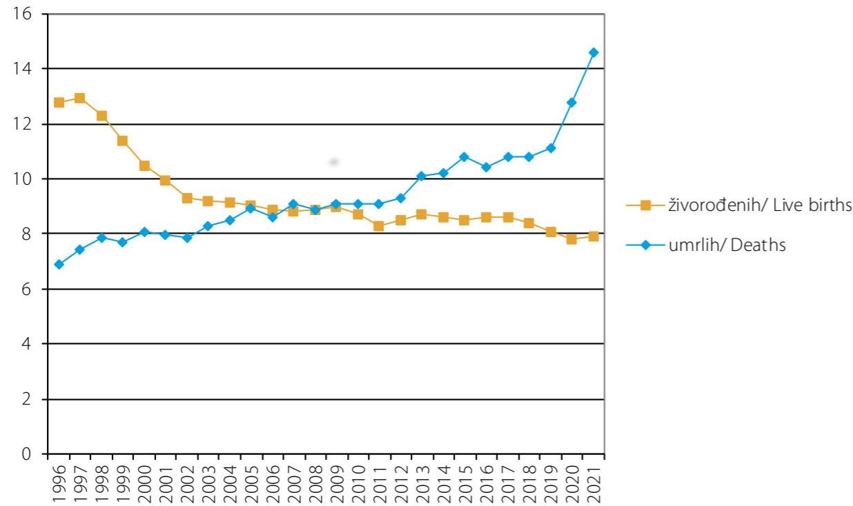
Grafikon 3. Stope prirodnog kretanja stanovništva Graph 3. Population natural change rates
