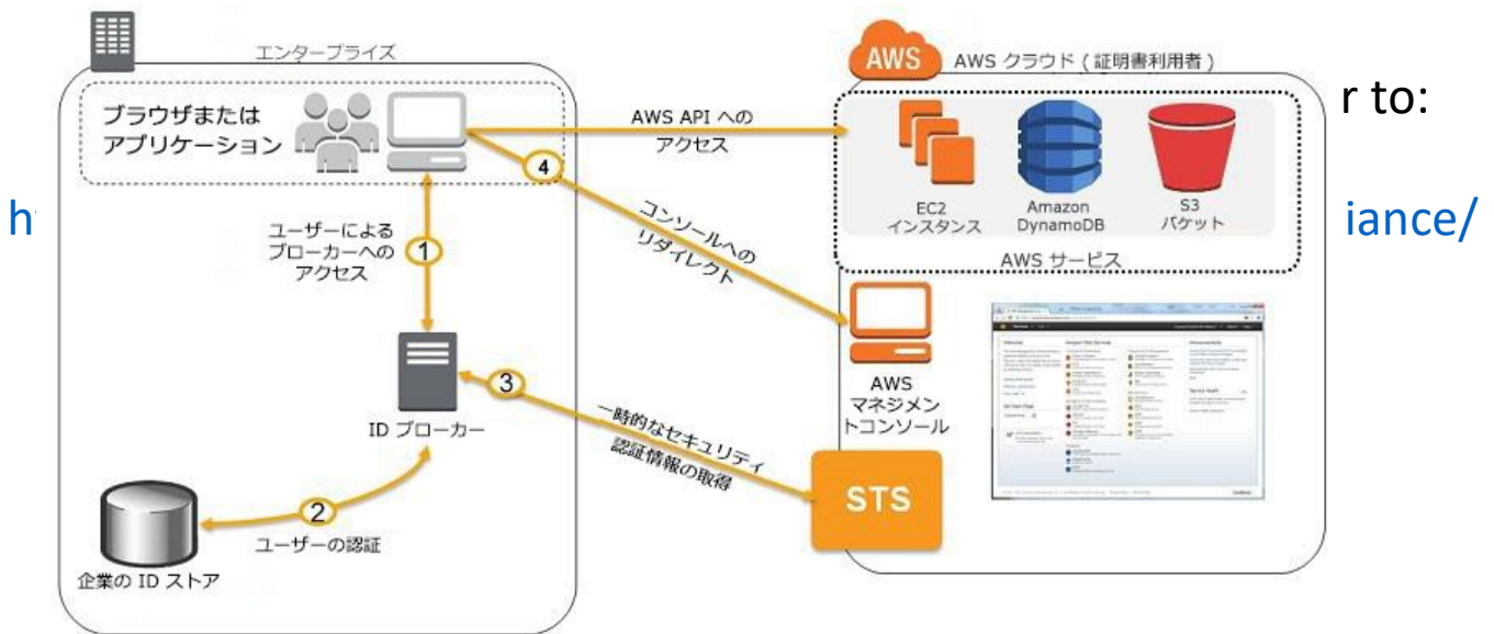
図 5:一時的なセキュリティ 認証情報を使用した AWS ID フェデレーション
