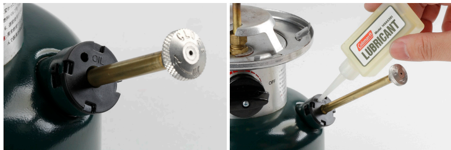
リユベリカントはポンプカップの「OIL」マークの隣にある穴から2～3滴ほど注入してください。
