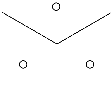
图 15.8: 最近邻算法如何将输入空间分成不同区域的图示。最近邻算法是一个基于非分布式表示的学习算法的示例。不同的非分布式算法可以具有不同的几何形状, 但是它们通常将输入空间分成区域, 每个区域具有不同的参数。非分布式方法的优点是, 给定足够的参数, 它能够拟合一个训练集, 而不需要复杂的优化算法。因为它直接为每个区域独立地设置不同的参数。缺点是, 非分布式表示的模型只能通过平滑先验来局部地泛化, 因此学习波峰波谷多于样本的复杂函数时, 该方法是不可行的。和分布式表示的对比, 可以参照图 15.7。
