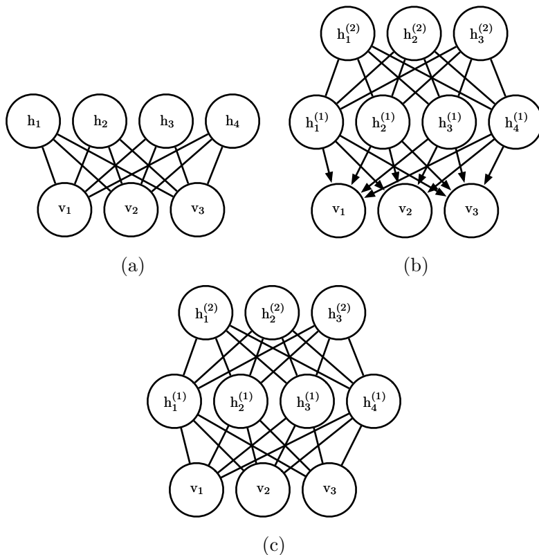
图 20.1: 可以用受限玻尔兹曼机构建的模型示例。(a)受限玻尔兹曼机本身是基于二分图的无向图模型,在图的一部分具有可见单元,另一部分具有隐藏单元。可见单元之间没有连接,隐藏单元之间也没有任何连接。通常每个可见单元连接到每个隐藏单元,但也可以构造稀疏连接的RBM,如卷积RBM。(b)深度信念网络是涉及有向和无向连接的混合图模型。与RBM一样,它也没有层内连接。然而,DBN具有多个隐藏层,因此隐藏单元之间的连接在分开的层中。深度信念网络所需的所有局部条件概率分布都直接复制RBM的局部条件概率分布。或者,我们也可以用完全无向图表示深度信念网络,但是它需要层内连接来捕获父节点间的依赖关系。(c)深度玻尔兹曼机是具有几层潜变量的无向图模型。与RBM和DBN一样,DBM也缺少层内连接。DBM与RBM的联系不如DBN紧密。当从RBM堆栈初始化DBM时,有必要对RBM的参数稍作修改。某些种类的DBM可以直接训练,而不用先训练一组RBM。
