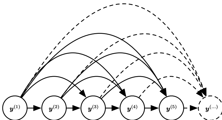
图 10.7: 序列 \mathbf{y}^{(1)}, \mathbf{y}^{(2)}, \dots, \mathbf{y}^{(t)}, \dots 的全连接图模型。给定先前的值，每个过去的观察值 \mathbf{y}^{(i)} 可以影响一些 \mathbf{y}^{(t)} (t > i) 的条件分布。当序列中每个元素的输入和参数的数目越来越多，根据此图直接参数化图模型（如式 (10.6) 中）可能是非常低效的。RNN 可以通过高效的参数化获得相同的全连接，如图 10.8 所示。
