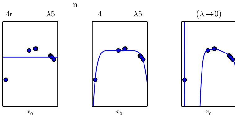
图 5.5: 我们使用高阶多项式回归模型来拟合图 5.2 中训练样本。真实函数是二次的, 但是在这里我们只使用 9 阶多项式。我们通过改变权重衰减的量来避免高阶模型的过拟合问题。(左) 当 \lambda 非常大时, 我们可以强迫模型学习到了一个没有斜率的函数。由于它只能表示一个常数函数, 所以会导致欠拟合。(中) 取一个适当的 \lambda 时, 学习算法能够用一个正常的形状来恢复曲率。即使模型能够用更复杂的形状来表示函数, 权重衰减鼓励用一个带有更小参数的更简单的模型来描述它。(右) 当权重衰减趋近于 0 (即使用 Moore-Penrose 伪逆来解决这个带有最小正则化的欠定问题) 时, 这个 9 阶多项式会导致严重的过拟合, 这和我们图 5.2 中看到的一样。
