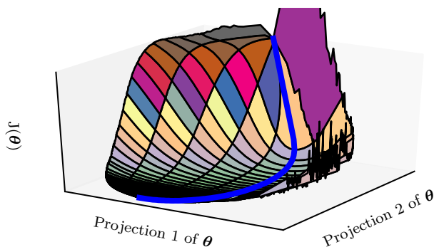
图 8.2: 神经网络代价函数的可视化。这些可视化对应用于真实对象识别和自然语言处理任务的前馈神经网络、卷积网络和循环网络而言是类似的。令人惊讶的是，这些可视化通常不会显示出很多明显的障碍。大约 2012 年，在随机梯度下降开始成功训练非常大的模型之前，相比这些投影所显示的神经网络代价函数的表面通常被认为有更多的非凸结构。该投影所显示的主要障碍是初始参数附近的高代价鞍点，但如由蓝色路径所示，SGD 训练轨迹能轻易地逃脱该鞍点。大多数训练时间花费在横穿代价函数中相对平坦的峡谷，可能由于梯度中的高噪声、或该区域中 Hessian 矩阵的病态条件，或者需要经过间接的弧路径绕过图中可见的高“山”。图经 Goodfellow et al. (2015) 许可改编。
