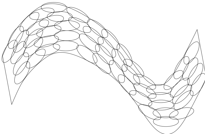
图 14.9: 如果每个位置处的切平面 (见图 14.6) 是已知的, 则它们可以平铺后形成全局坐标系或密度函数。每个局部块可以被认为是局部欧几里德坐标系或者是局部平面高斯或“薄饼”, 在与薄饼正交的方向上具有非常小的方差而在定义坐标系的方向上具有非常大的方差。这些高斯的混合提供了估计的密度函数, 如流形中的 Parzen 窗口算法 (Vincent and Bengio, 2003) 或其非局部的基于神经网络的变体 (Bengio et al. , 2006b)。
