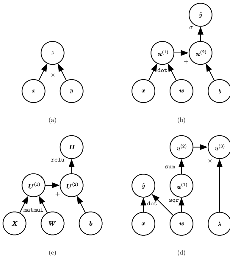
图 6.8: 一些计算图的示例。(a) 使用 \times 操作计算 z = xy 的图。(b) 用于逻辑回归预测 \hat{y} = \sigma(\mathbf{x}^\top \mathbf{w} + b) 的图。一些中间表达式在代数表达式中没有名称，但在图形中却需要。我们简单地将第 i 个这样的变量命名为 \mathbf{u}^{(i)} 。(c) 表达式 \mathbf{H} = \max\{0, \mathbf{X}\mathbf{W} + \mathbf{b}\} 的计算图，在给定包含小批量输入数据的设计矩阵 \mathbf{X} 时，它计算整流线性单元激活的设计矩阵 \mathbf{H} 。(d) 示例 a-c 对每个变量最多只实施一个操作，但是对变量实施多个操作也是可能的。这里我们展示一个计算图，它对线性回归模型的权重 \mathbf{w} 实施多个操作。这个权重不仅用于预测 \hat{y} ，也用于权重衰减罚项 \lambda \sum_i w_i^2 。
