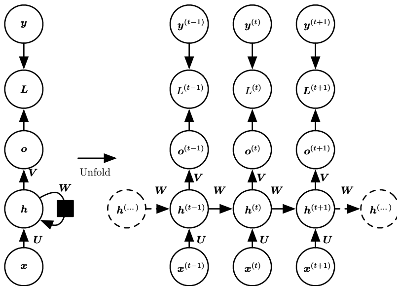
图 10.3: 计算循环神经网络(将 x 值的输入序列映射到输出值 o 的对应序列) 训练损失的计算图。损失 L 衡量每个 o 与相应的训练目标 y 的距离。当使用 softmax 输出时, 我们假设 o 是未归一化的对数概率。损失 L 内部计算 \hat{y} = \text{softmax}(o) , 并将其与目标 y 比较。RNN 输入到隐藏的连接由权重矩阵 U 参数化, 隐藏到隐藏的循环连接由权重矩阵 W 参数化以及隐藏到输出的连接由权重矩阵 V 参数化。式 (10.8) 定义了该模型中的前向传播。(左) 使用循环连接绘制的 RNN 和它的损失。(右) 同一网络被视为展开的计算图, 其中每个节点现在与一个特定的时间实例相关联。
