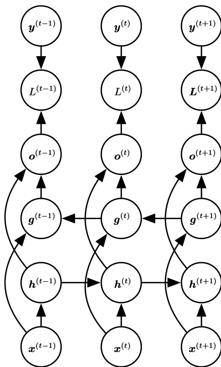
图 10.11: 典型的双向循环神经网络中的计算, 意图学习将输入序列 \mathbf{x} 映射到目标序列 \mathbf{y} (在每个步骤 t 具有损失 L^{(t)} )。循环性 \mathbf{h} 在时间上向前传播信息 (向右), 而循环性 \mathbf{g} 在时间上向后传播信息 (向左)。因此在每个点 t , 输出单元 \mathbf{o}^{(t)} 可以受益于输入 \mathbf{h}^{(t)} 中关于过去的相关概要以及输入 \mathbf{g}^{(t)} 中关于未来的相关概要。
