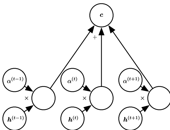
图 12.6: 由 Bahdanau et al. (2015) 引入的现代注意力机制, 本质上是加权平均。注意力机制对具有权重 \alpha^{(t)} 的特征向量 h^{(t)} 进行加权平均形成上下文向量 c 。在一些应用中, 特征向量 h 是神经网络的隐藏单元, 但它们也可以是模型的原始输入。权重 \alpha^{(t)} 由模型本身产生。它们通常是区间 [0, 1] 中的值, 并且旨在仅仅集中在单个 h^{(t)} 周围, 使得加权平均精确地读取接近一个特定时间步的特征向量。权重 \alpha^{(t)} 通常由模型另一部分发出的相关性得分应用 softmax 函数后产生。注意力机制在计算上需要比直接索引期望的 h^{(t)} 付出更高的代价, 但直接索引不能使用梯度下降训练。基于加权平均的注意力机制是平滑、可微的近似, 可以使用现有优化算法训练。
