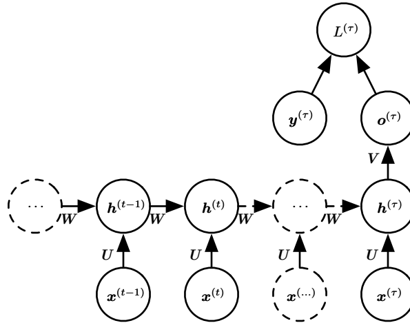
图 10.5: 关于时间展开的循环神经网络, 在序列结束时具有单个输出。这样的网络可以用于概括序列并产生用于进一步处理的固定大小的表示。在结束处可能存在目标 (如此处所示), 或者通过更下游模块的反向传播来获得输出 o^{(t)} 上的梯度。
