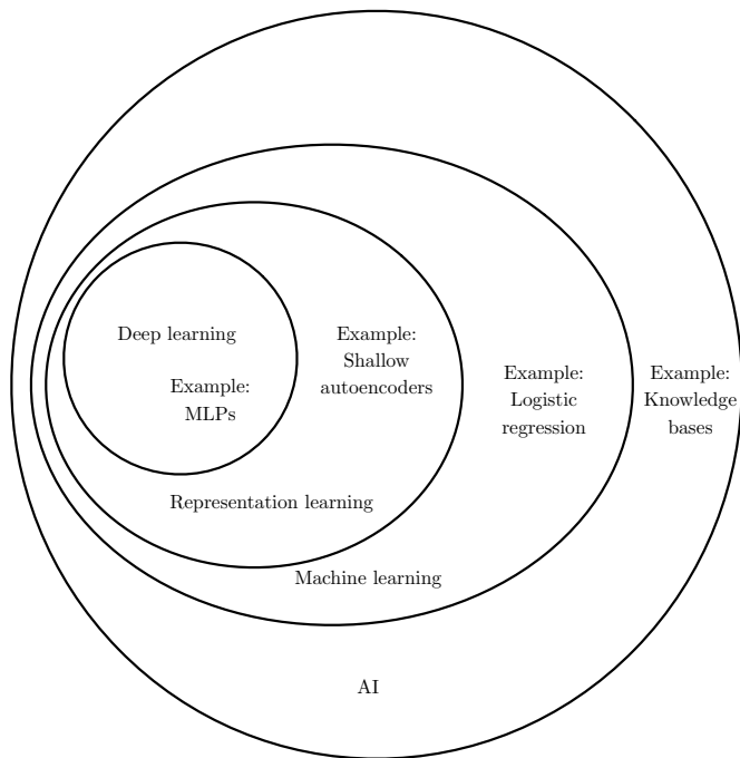
图 1.4: 维恩图展示了深度学习是一种表示学习,也是一种机器学习,可以用于许多(但不是全部) AI 方法。维恩图的每个部分包括一个 AI 技术的示例。
