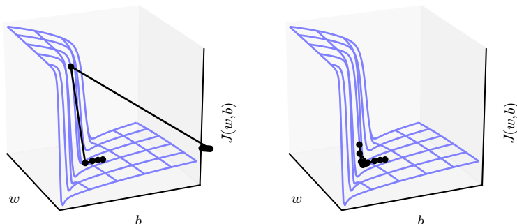
图 10.17: 梯度截断在有两个参数 w 和 b 的循环网络中的效果示例。梯度截断可以使梯度下降在极陡峭的悬崖附近更合理地执行。这些陡峭的悬崖通常发生在循环网络中，位于循环网络近似线性的附近。悬崖在时间步的数量上呈指数地陡峭，因为对于每个时间步，权重矩阵都自乘一次。(左) 没有梯度截断的梯度下降越过这个小峡谷的底部，然后从悬崖面接收非常大的梯度。大梯度灾难性地将参数推到图的轴外。(右) 使用梯度截断的梯度下降对悬崖的反应更温和。当它上升到悬崖面时，步长受到限制，使得它不会被推出靠近解的陡峭区域。经 Pascanu et al. (2013a) 许可可改编此图。
