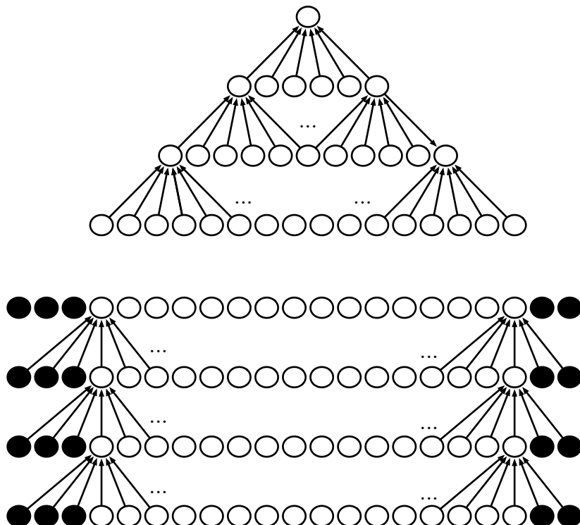
图 9.13: 零填充对网络大小的影响。考虑一个卷积网络, 每层有一个宽度为六的核。在这个例子中, 我们不使用任何池化, 所以只有卷积操作本身缩小网络的大小。(上) 在这个卷积网络中, 我们不使用任何隐含的零填充。这使得表示在每层缩小五个像素。从十六个像素的输入开始, 我们只能有三个卷积层, 并且最后一层不能移动核, 所以可以说只有两层是真正的卷积层。可以通过使用较小的核来减缓收缩速率, 但是较小的核表示能力不足, 并且在这种结构中一些收缩是不可避免的。(下) 通过向每层添加五个隐含的零, 我们防止了表示随深度收缩。这允许我们设计一个任意深的卷积网络。
