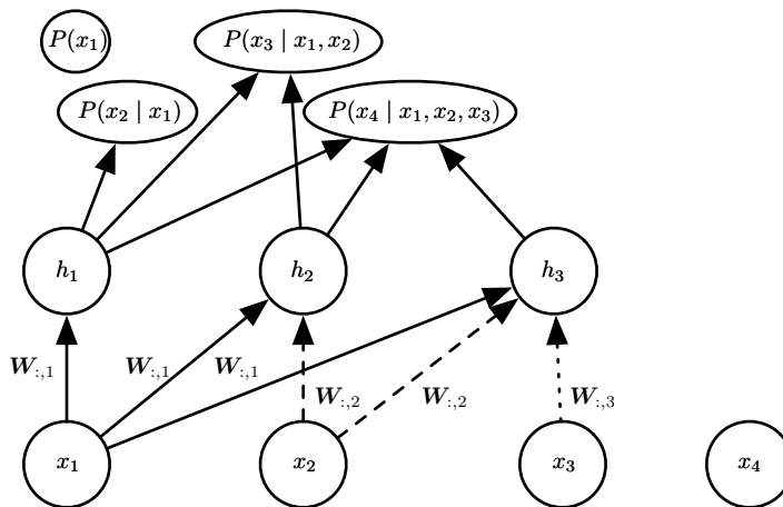
图 20.10: 神经自回归密度估计器 (NADE) 的示意图。隐藏单元被组织在组 h^{(j)} 中, 使得只有输入 x_1, \dots, x_i 参与计算 h^{(i)} 和预测 P(x_j | x_{j-1}, \dots, x_1) (对于 j > i )。NADE 使用特定的权重共享模式区别于早期的神经自回归网络: W'_{j,k,i} = W_{k,i} 被共享于所有从 x_i 到任何 j \geq i 组中第 k 个单元的权重 (在图中使用相同的线型表示复制权重的每个实例)。注意向量 (W_{1,i}, W_{2,i}, \dots, W_{n,i}) 记为 W_{:,i} 。
