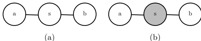
图 16.6: (a) 随机变量 a 和随机变量 b 之间穿过 s 的路径是活跃的，因为 s 是观察不到的。这意味着 a, b 之间不是分离的。(b) 图中 s 用阴影填充，表示它是可观察的。因为 a 和 b 之间的唯一路径通过 s ，并且这条路径是不活跃的，我们可以得出结论，在给定 s 的条件下 a 和 b 是分离的。
