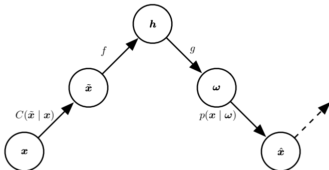
图 20.11: 马尔可夫链的每个步骤与训练好的去噪自编码器相关联, 根据由去噪对数似然准则隐式训练的概率模型生成样本。每个步骤包括: (a) 通过损坏过程 C 向状态 \mathbf{x} 注入噪声产生 \tilde{\mathbf{x}} , (b) 用函数 f 对其编码, 产生 \mathbf{h} = f(\tilde{\mathbf{x}}) , (c) 用函数 g 解码结果, 产生用于重构分布的参数 \omega , (d) 给定 \omega , 从重构分布 p(\mathbf{x} | \omega = g(f(\tilde{\mathbf{x}}))) 采样新状态。在典型的平方重构误差情况下, g(\mathbf{h}) = \hat{\mathbf{x}} , 并估计 \mathbb{E}[\mathbf{x} | \tilde{\mathbf{x}}] , 损坏包括添加高斯噪声, 并且从 p(\mathbf{x} | \omega) 的采样包括第二次向重构 \hat{\mathbf{x}} 添加高斯噪声。后者的噪声水平应对应于重构的均方误差, 而注入的噪声是控制混合速度以及估计器平滑经验分布程度的超参数 (Vincent, 2011)。在这所示的例子中, 只有 C 和 p 条件是随机步骤 ( f 和 g 是确定性计算), 我们也可以在自编码器内部注入噪声, 如生成随机网络 (Bengio et al. , 2014)。
