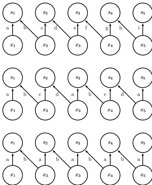
图 9.16: 局部连接层、平铺卷积和标准卷积的比较。当使用相同大小的核时,这三种方法在单元之间具有相同的连接。此图是对使用两个像素宽的核的说明。这三种方法之间的区别在于它们如何共享参数。(上)局部连接层根本没有共享参数。我们对每个连接使用唯一的字母标记,来表明每个连接都有它自身的权重。(中)平铺卷积有 t 个不同的核。这里我们说明 t = 2 的情况。其中一个核具有标记为“a”和“b”的边,而另一个具有标记为“c”和“d”的边。每当我们在输出中右移一个像素后,我们使用一个不同的核。这意味着,与局部连接层类似,输出中的相邻单元具有不同的参数。与局部连接层不同的是,在我们遍历所有可用的 t 个核之后,我们循环回到了第一个核。如果两个输出单元间隔 t 个步长的倍数,则它们共享参数。(下)传统卷积等效于 t = 1 的平铺卷积。它只有一个核,并且被应用到各个地方,我们在图中表示为在各处使用具有标记为“a”和“b”的边的核。
