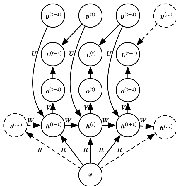
图 10.9: 将固定长度的向量 \mathbf{x} 映射到序列 \mathbf{Y} 上分布的 RNN。这类 RNN 适用于很多任务如图注, 其中单个图像作为模型的输入, 然后产生描述图像的词序列。观察到的输出序列的每个元素 \mathbf{y}^{(t)} 同时用作输入 (对于当前时间步) 和训练期间的目标 (对于前一时间步)。
