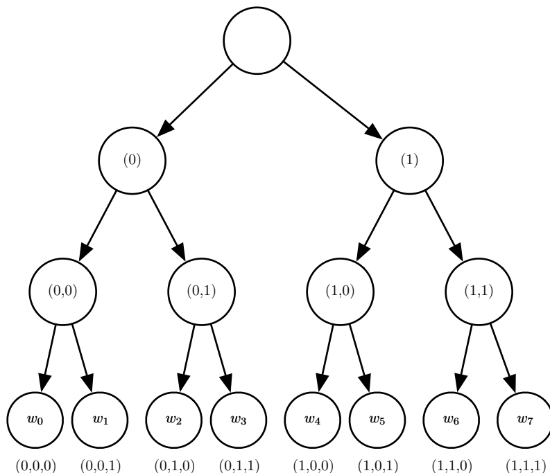
图 12.4: 词类别简单层次结构的示意图, 其中 8 个词 w_0, \dots, w_7 组织成三级层次结构。树的叶子表示实际特定的词。内部节点表示词的组别。任何节点都可以通过二值决策序列 (0=左, 1=右) 索引, 从根到达节点。超类 (0) 包含类 (0,0) 和 (0,1), 其中分别包含词 \{w_0, w_1\} 和 \{w_2, w_3\} 的集合, 类似地超类 (1) 包含类 (1,0) 和 (1,1), 分别包含词 \{w_4, w_5\} 和 \{w_6, w_7\} 。如果树充分平衡, 则最大深度 (二值决策的数量) 与词数 |\mathcal{V}| 的对数同阶: 从 |\mathcal{V}| 个词中选一个词只需执行 \mathcal{O}(\log |\mathcal{V}|) 次操作 (从根开始的路径上的每个节点一次操作)。在该示例中, 我们乘三次概率就能计算词 y 的概率, 这三次概率与从根到节点 y 的路径上每个节点向左或向右的二值决策相关联。令 b_i(y) 为遍历树移向 y 时的第 i 个二值决策。对输出 y 进行采样的概率可以通过条件概率的链式法则分解为条件概率的乘积, 其中每个节点由这些位的前缀索引。例如, 节点 (1,0) 对应于前缀 (b_0(w_4) = 1, b_1(w_4) = 0) , 并且 w_4 的概率可以如下分解:
