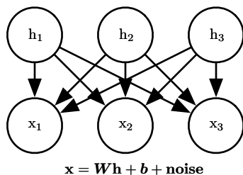
图 13.1: 描述线性因子模型族的有向图模型, 其中我们假设观察到的数据向量 \mathbf{x} 是通过独立的潜在因子 \mathbf{h} 的线性组合再加上一定噪声获得的。不同的模型, 比如概率 PCA, 因子分析或者是 ICA, 都是选择了不同形式的噪声以及先验 p(\mathbf{h}) 。
