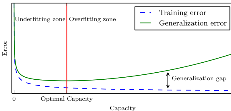
图 5.3: 容量和误差之间的典型关系。训练误差和测试误差表现得非常不同。在图的左端，训练误差和泛化误差都非常高。这是欠拟合机制（underfitting regime）。当我们增加容量时，训练误差减小，但是训练误差和泛化误差之间的间距却不断扩大。最终，这个间距的大小超过了训练误差的下降，我们进入到了过拟合机制（overfitting regime），其中容量过大，超过了最佳容量（optimal capacity）。
