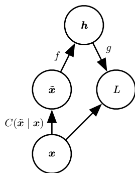
图 14.3: 去噪自编码器代价函数的计算图。去噪自编码器被训练为从损坏的版本 \tilde{\mathbf{x}} 重构干净数据点 \mathbf{x} 。这可以通过最小化损失 L = -\log p_{\text{decoder}}(\mathbf{x} | \mathbf{h} = f(\tilde{\mathbf{x}})) 实现,其中 \tilde{\mathbf{x}} 是样本 \mathbf{x} 经过损坏过程 C(\tilde{\mathbf{x}} | \mathbf{x}) 后得到的损坏版本。通常,分布 p_{\text{decoder}} 是因子的分布(平均参数由前馈网络 g 给出)。
