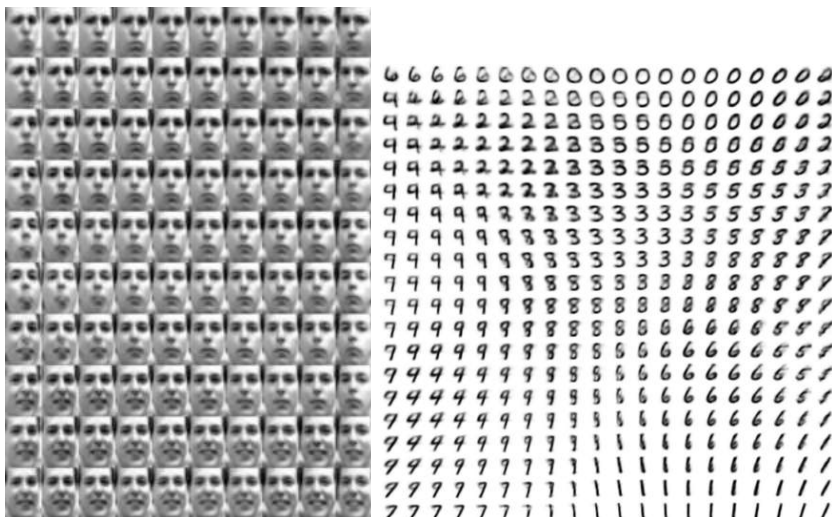
图 20.6: 由变分自编码器学习的高维流形在 2 维坐标系中的示例 (Kingma and Welling, 2014a)。我们可以在纸上直接绘制两个可视化的维度，因此可以使用 2 维潜在编码训练模型来了解模型的工作原理（即使我们认为数据流形的固有维度要高得多）。图中所示的图像不是来自训练集的样本，而是仅仅通过改变 2 维“编码” z ，由模型 p(x|z) 实际生成的图像 x （每个图像对应于“编码” z 位于 2 维均匀网格的不同选择）。(左) Frey 人脸流形的 2 维映射。其中一个维度（水平）已发现大致对应于面部的旋转，而另一个（垂直）对应于情绪表达。(右) MNIST 流形的 2 维映射。
