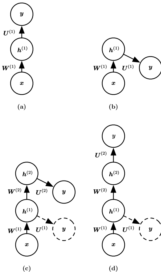
图 8.7: 一种形式的贪心监督预训练的示意图 (Bengio et al. , 2007a)。(a) 我们从训练一个足够浅的架构开始。(b) 同一个架构的另一描绘。(c) 我们只保留原始网络的输入到隐藏层, 并丢弃隐藏到输出层。我们将第一层隐藏层的输出作为输入发送到另一监督单隐层 MLP (使用与第一个网络相同的目标训练), 从而可以添加第二层隐藏层。这可以根据需要重复多层。(d) 所得架构的另一种描绘, 可视为前馈网络。为了进一步改进优化, 我们可以联合地精调所有层 (仅在该过程的结束或者该过程的每个阶段)。
