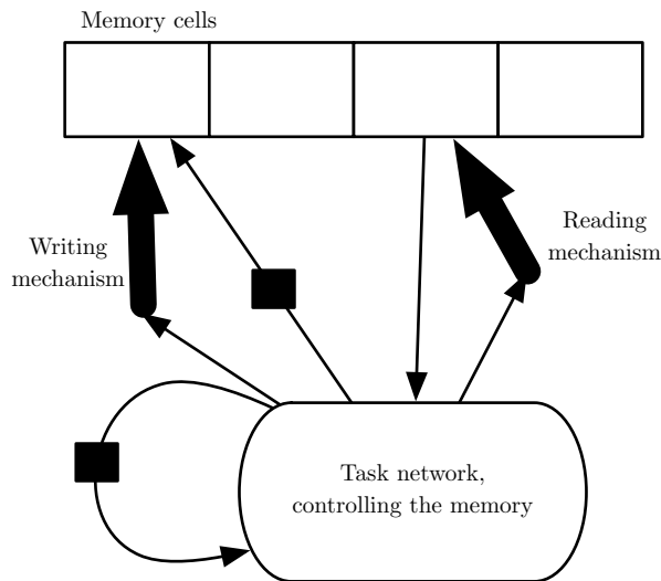
图 10.18: 具有外显记忆网络的示意图，具备神经网络图灵机的一些关键设计元素。在此图中，我们将模型的“表示”部分（“任务网络”，这里是底部的循环网络）与存储事实的模型（记忆单元的集合）的“存储器”部分区分开。任务网络学习“控制”存储器，决定从哪读取以及在哪写入（通过读取和写入机制，由指向读取和写入地址的粗箭头指示）。
