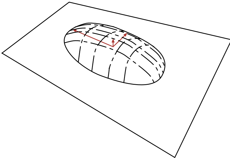
图 13.3: 平坦的高斯能够描述一个低维流形附近的概率密度。此图表示了“流形平面”上“馅饼”的上半部分, 并且这个平面穿过了馅饼的中心。正交于流形方向(指向平面外的箭头方向)的方差非常小, 可以被看作是“噪声”, 其他方向(平面内的箭头)的方差则很大, 对应了“信号”以及降维数据的坐标系统。
