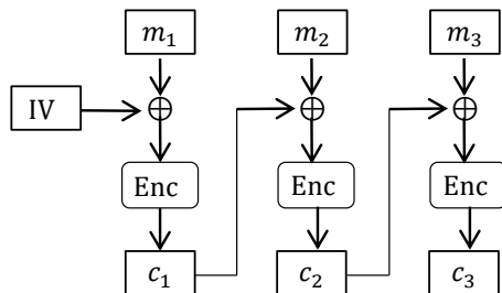
図 1.2 CBC モードの暗号化
