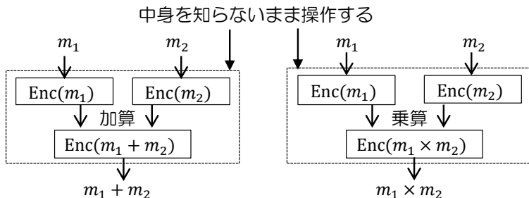
図 13.1 準同型暗号
