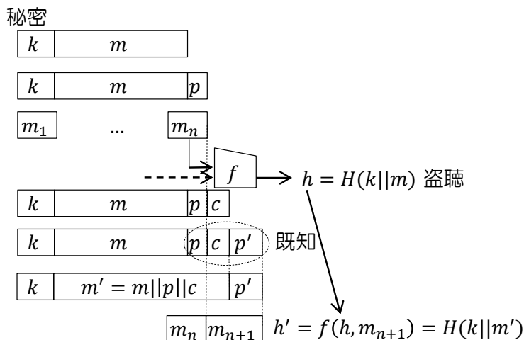
図 4.4 伸長攻撃
