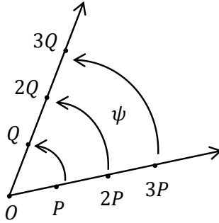
図 7.6 distortion 写像
