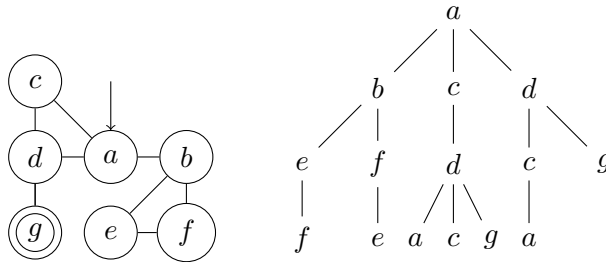
図 3.3: 探索木
