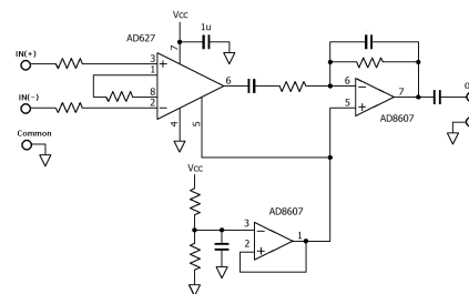
図 3 新しい筋電センシング回路の例と実験基板の外観
