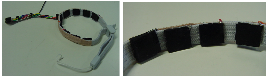
図 5 導電ゴムシート電極による筋電ベルトの外観(左)と電極のアップ(右)
