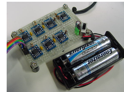
図 3 新しい筋電センシング回路の例と実験基板の外観
