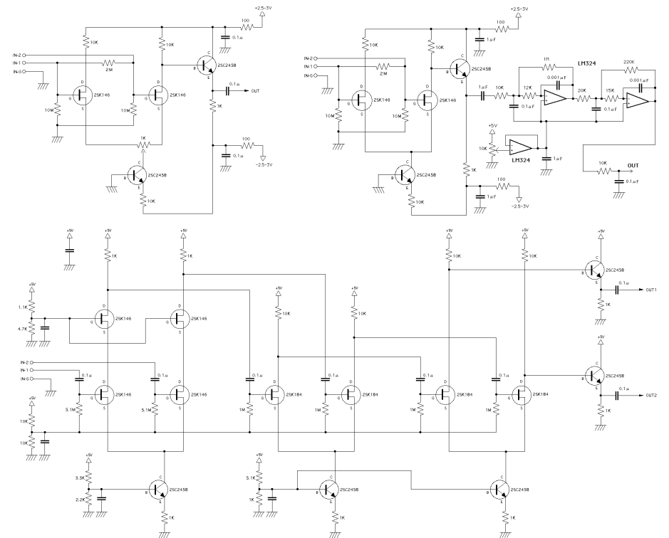
図 2 過去に採用してきた筋電センシング回路の例
