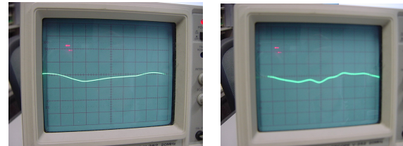
図 7 純銀円盤電極の出力信号例：脱力(左) 力を入れる(右)
