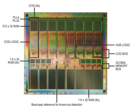
Fig.11 "Propeller"のチップ写真
