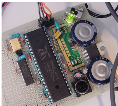
Fig.12 Propeller実験ボード
