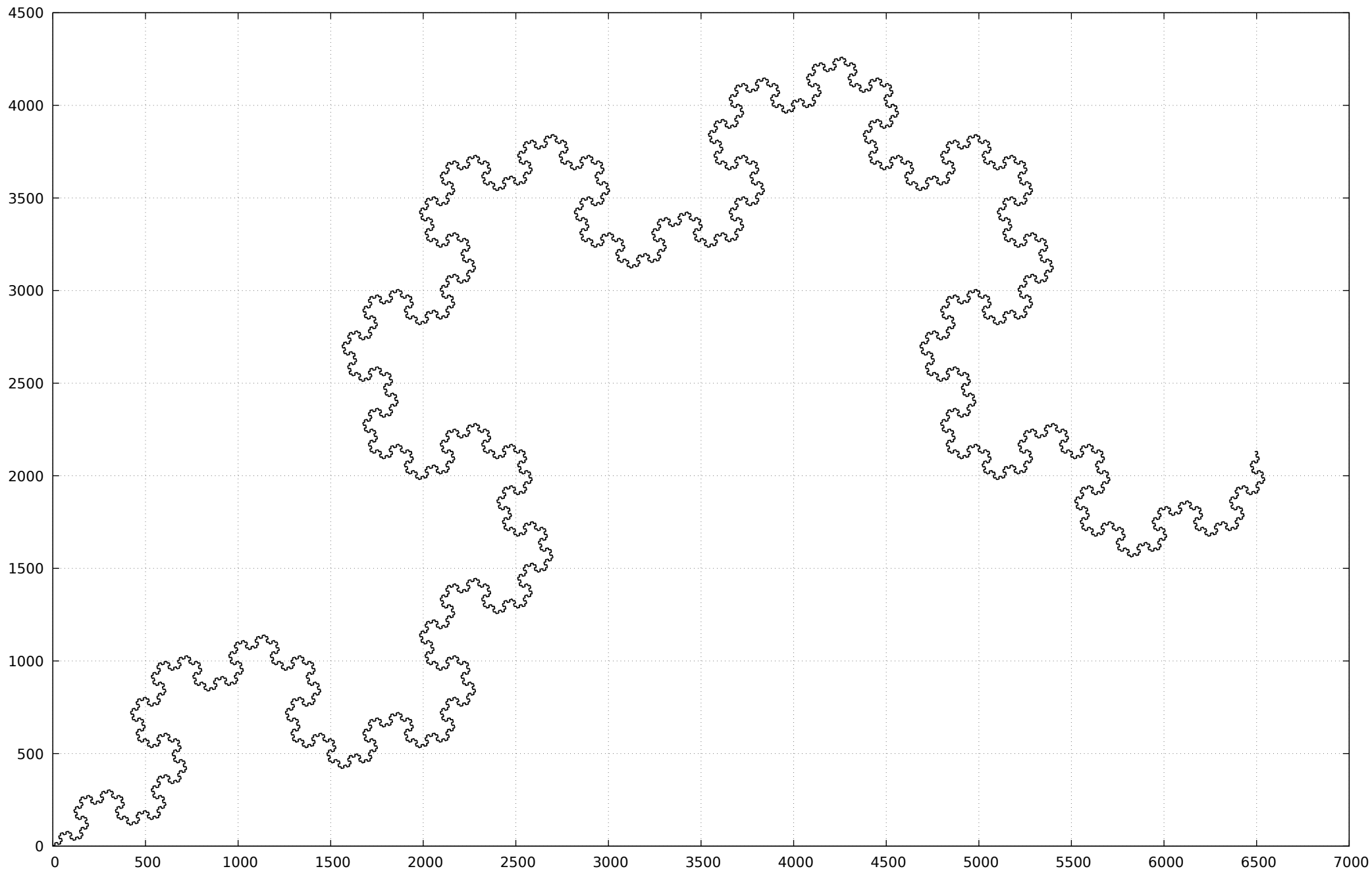
A307447 vs A307446 (n=1...50000)
