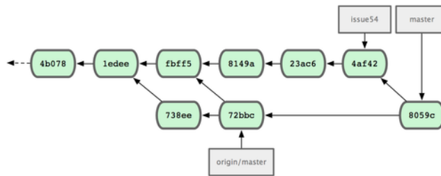
図 5.9: John の変更をマージした後の Jessica の履歴
