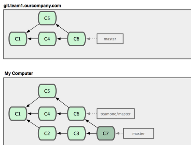
図 3.37: さらにコミットを取得し、作業環境にマージした状態
