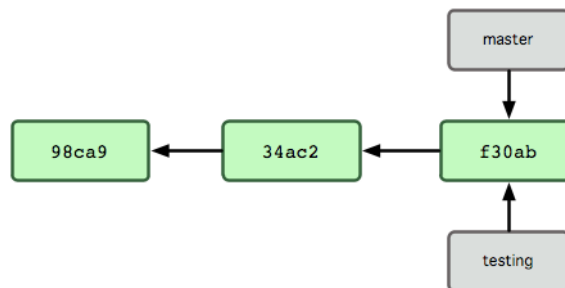
図 3.4: 複数のブランチがコミットデータの履歴を指す例
