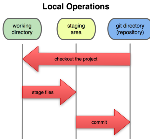
図 1.6: 作業ディレクトリ、ステージング・エリア、Gitディレクトリ
