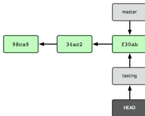
図 3.6: ブランチを切り替えると、HEAD の指す先が移動する
