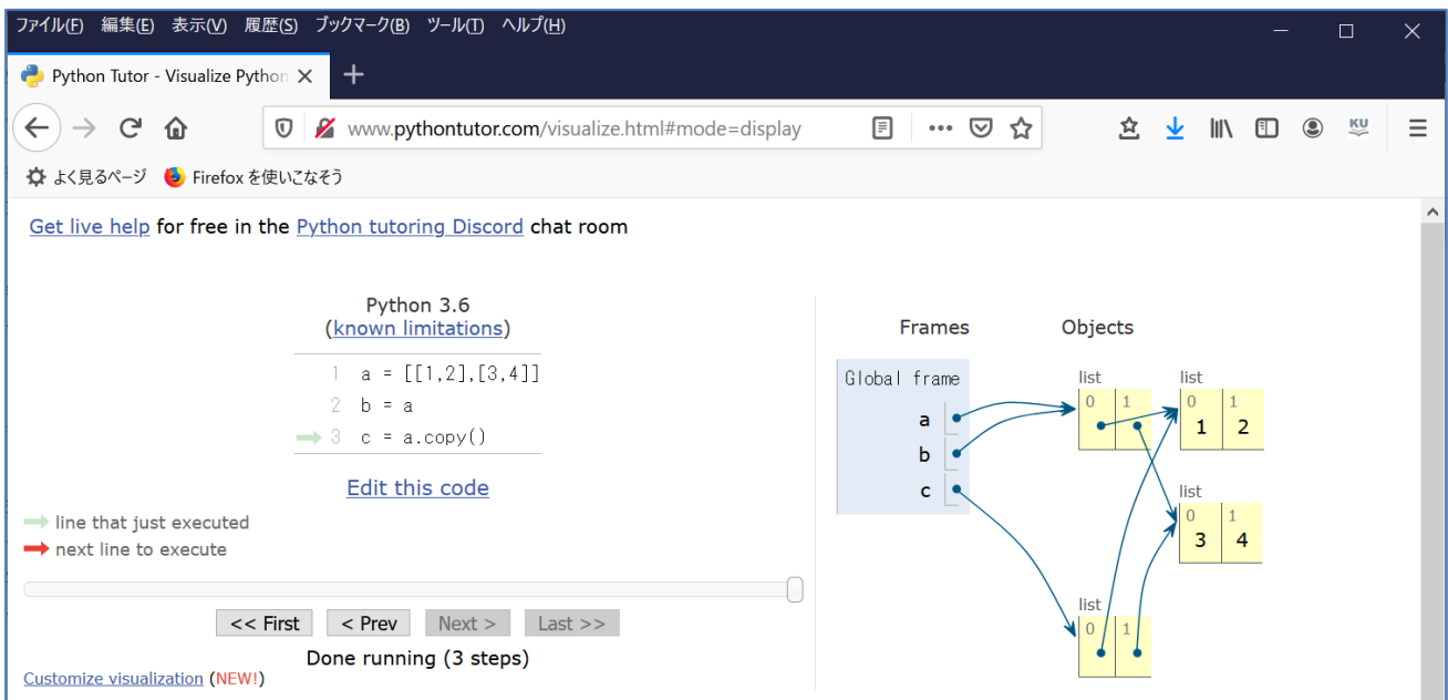
図 4-3 Python Tutor でリストの動作を確認する
