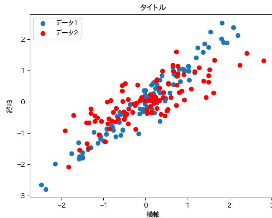
図 14-3 散布図の描画
