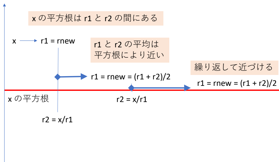
図 3-4 平方根の近似計算の直感的説明
