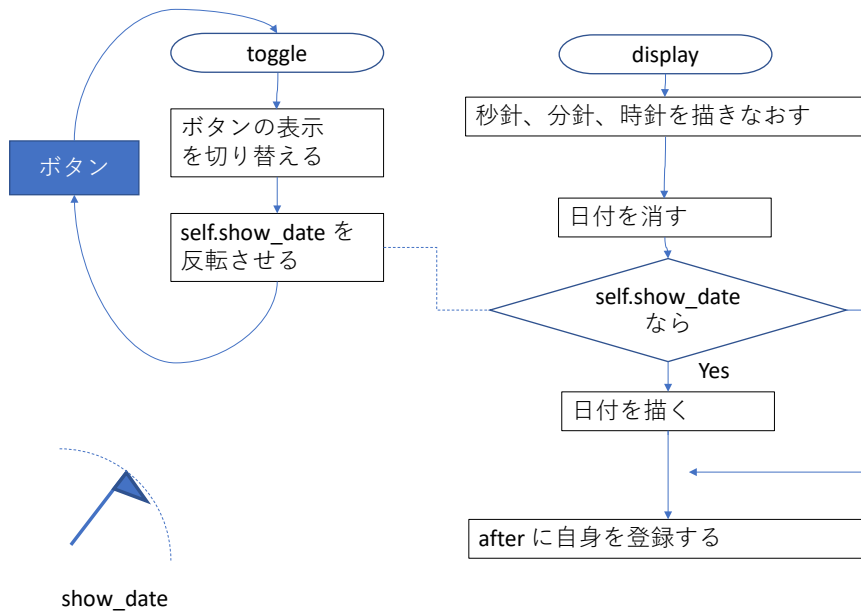
図 10-4 変数を介した動作の協調
