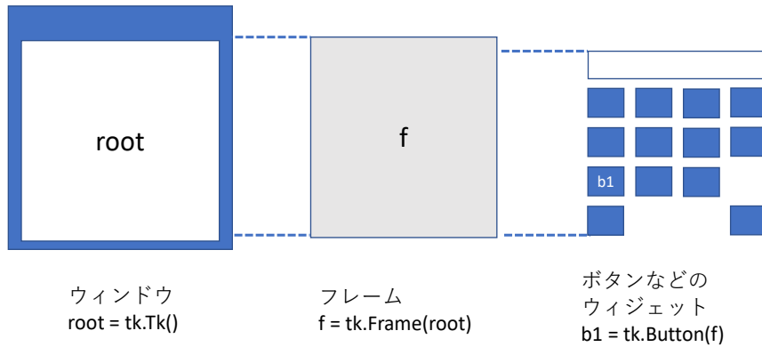
図 9-4 tkinter でのオブジェクトの関係
