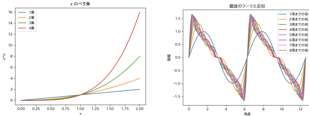
図 14-7 べき乗のグラフとこのぎり波の三角関数の和での近似
