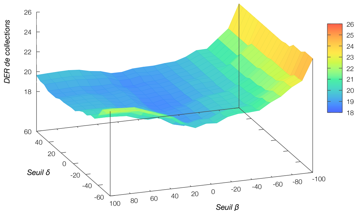
Figure 5.18 – Surface représentant le taux DER_{de\ collections} moyen obtenu en fonction des seuils \beta et \delta sur les 6 collections de niveau programme étudiées pour l'approche CC+HAC.
