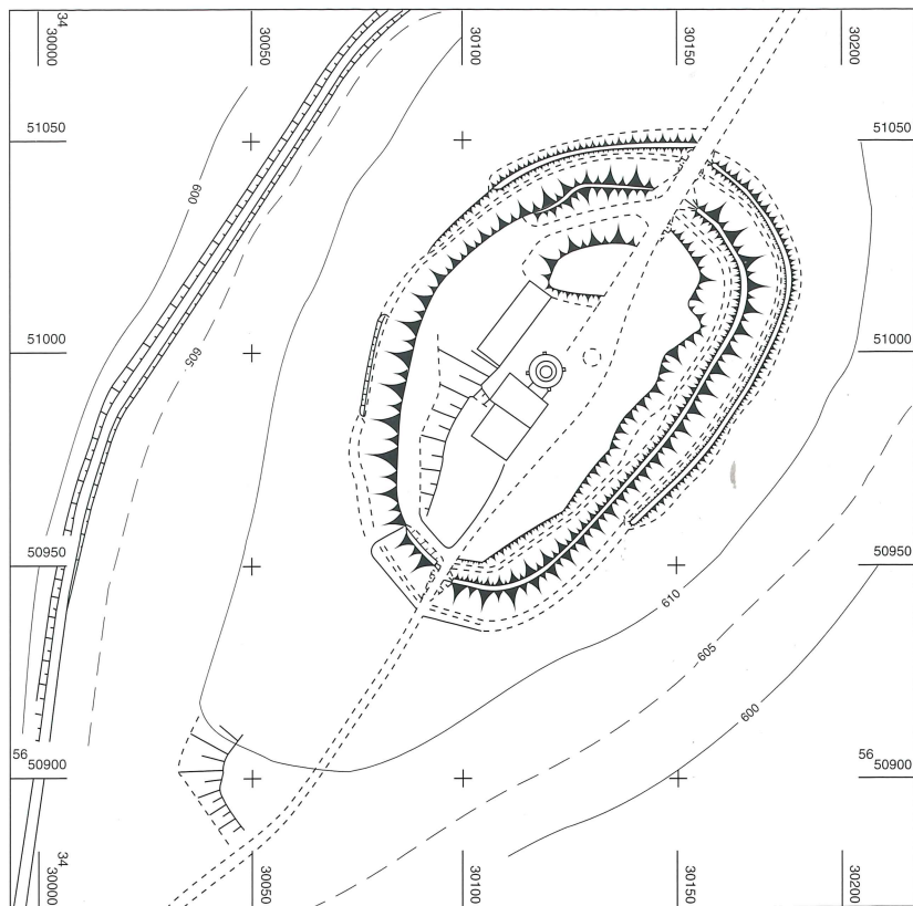
5 Grundriß des Kindelsberges. Maßstab ca. 1:2000 (Aufnahme Westf. Museum für Archäologie, Münster).
