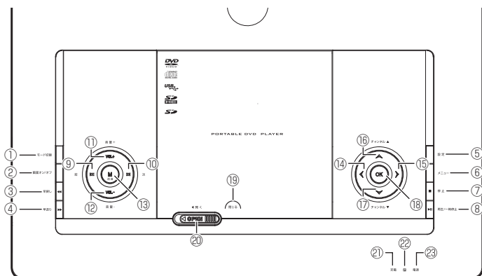
上面図
