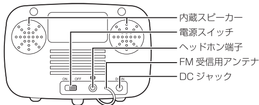
右側面
