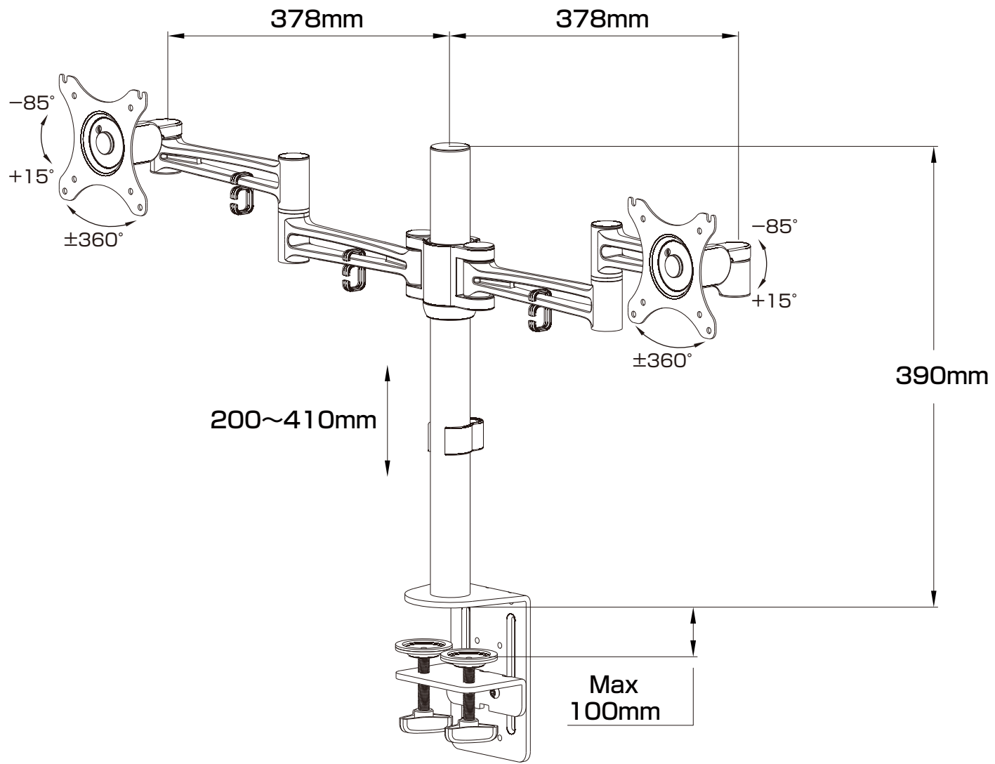
GH-AMCF02 外形寸法図
