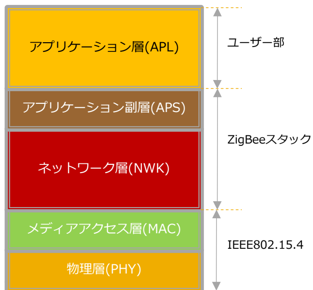
図1 ZigBee基本モデル
