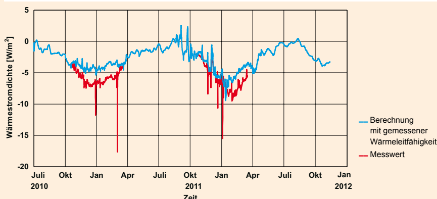
Diagramm 1: Berechneter zeitlicher Verlauf der Wärmestromdichte durch die Perimeterdämmung im Vergleich zu den Messwerten.
