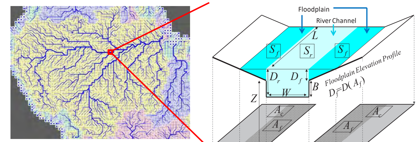
流域スケールでの水収支を表現する河道網
