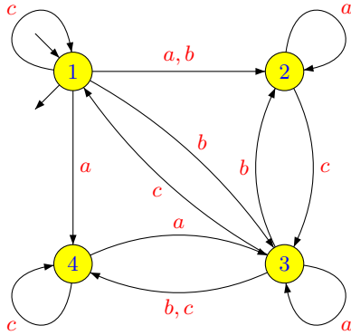
Figure 4.11. A nondeterministic automaton.
