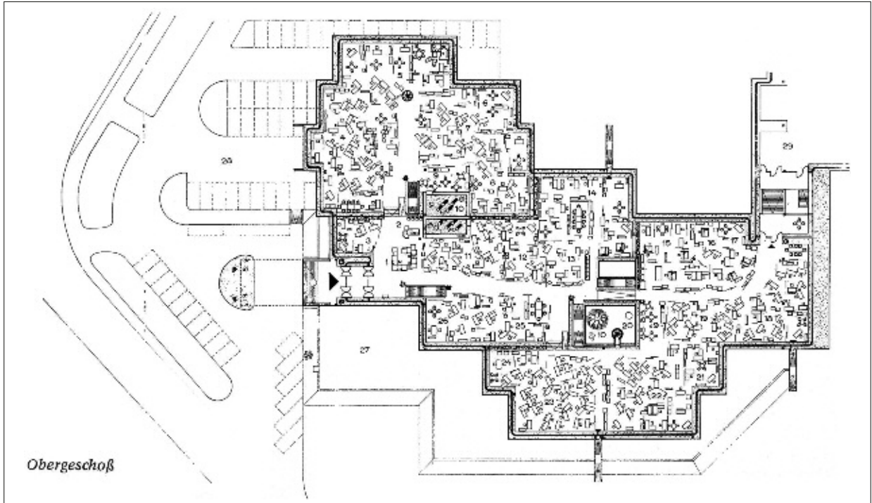
9 Herten, Herta AG, erbaut 1971. Architekt Werner Ruhbau, Grundrissorganisation der Bürolandschaft 1971.
