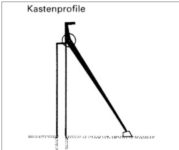
11 Statisches System des Fördergerüsts des Konrad-Ende-Schachtes.
