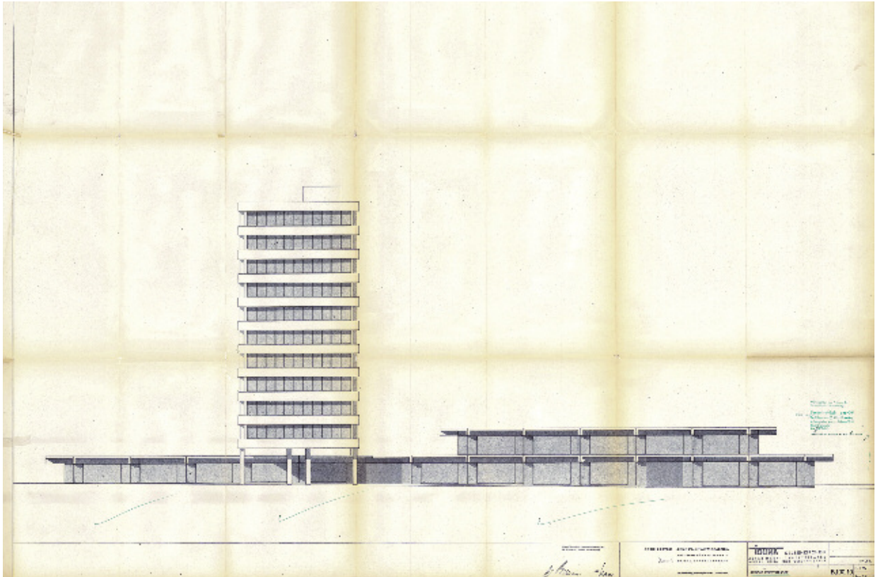
3 Gelsenkirchen, Iduna-Haus, erbaut 1966–1968. Architekten Friedrich Wilhelm Kraemer, Ernst Sieverts und Günter Pfennig. Ausführungsplanung 1966.
