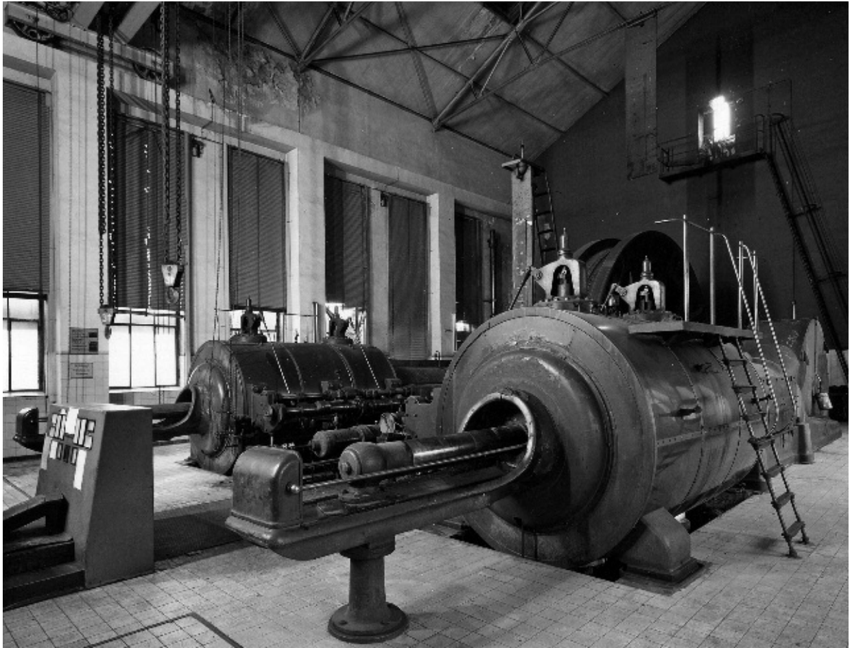
10 Dampfmachine des „Konrad Ende“-Schachtes, Zeche Recklinghausen II in Recklinghausen-Hochlarmark. 1989.
