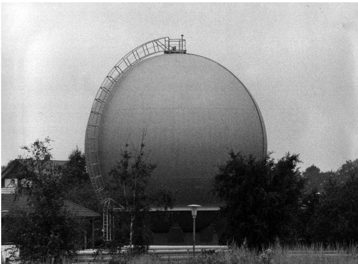
14 Kugelgasbehälter Gütersloh. 1981.
