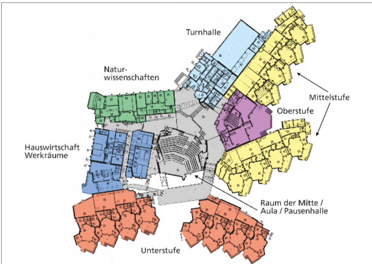
5 Marl, Scharounschule, ursprüngliche Nutzungen.
