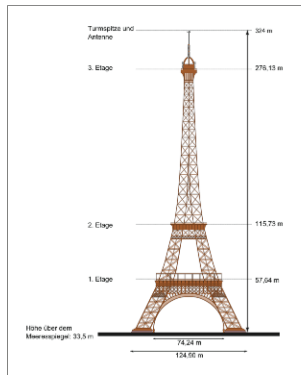
4 Schematische Zeichnung des Eiffelturms mit technischen Daten.
