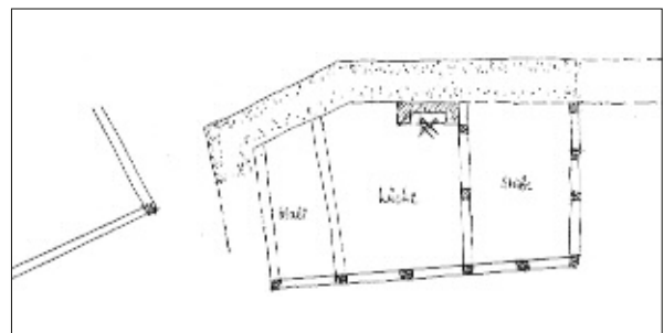
7 Iserlohn, Südengraben 28. Grundriss mit Angaben der ursprünglichen Raumfunktion. Skizze zum ursprünglichen Zustand des Mauerhauses um 1767 auf der Grundlage der baugeschichtlichen Untersuchung 2016.
