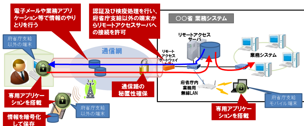
図 8.2.1-3 ファイル暗号化等セキュリティ機能を持つアプリケーションを活用したシステム構成例
