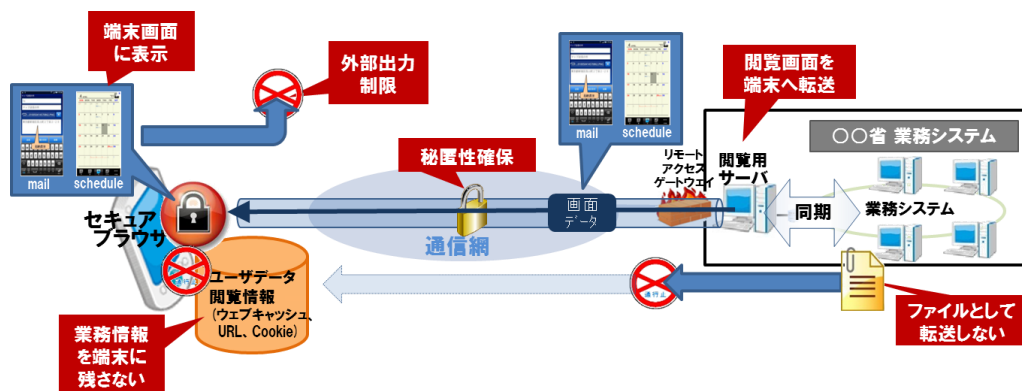
図 8.2.1-2 セキュアブラウザ活用型ソリューションのシステム構成例
