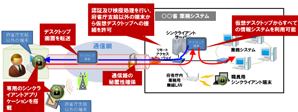
図 8.2.1-1 シンククライアントのシステム構成例
