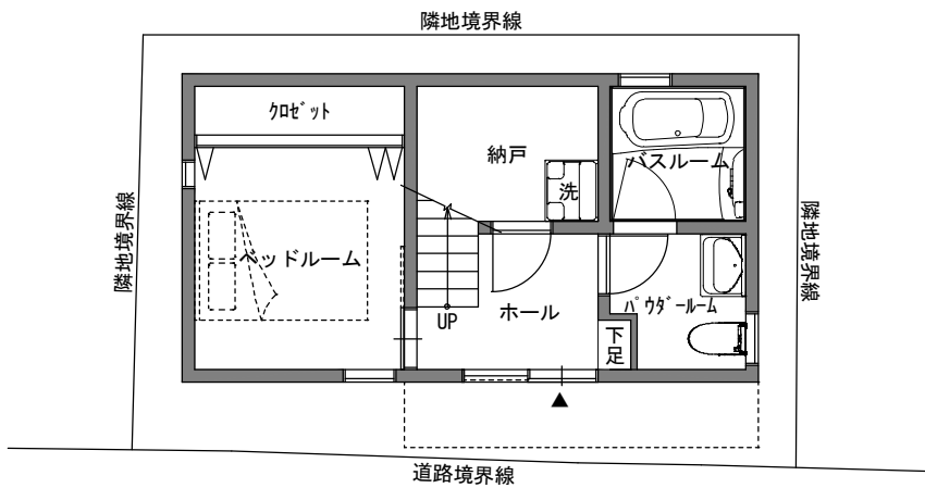
1階平面図 1/100
