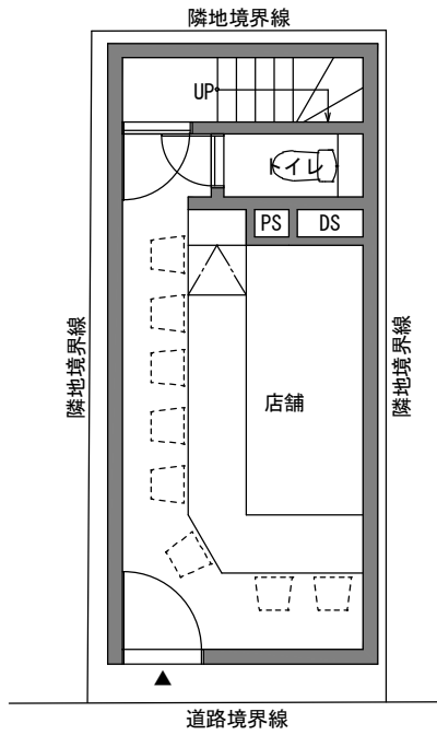
1 階平面図 1/100
