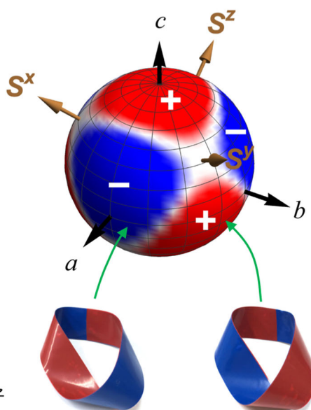
図 2 : (左) 通常の量子ホール効果状態とキタエフ量子スピン液体における半整数熱量子ホール効果状態のイメージ図。通常の量子ホール効果では、エッジ流は電子により運ばれる。その起源は電子の円運動（サイクロトロン運動）である。一方、キタエフ量子スピン液体においてエッジ流はマヨラナ粒子により運ばれる。 (右) 理論模型による半整数熱量子ホール効果の符号の角度依存性。正と負の符号はマヨラナ粒子がそれぞれ右ひねりと左ひねりのメビウスの輪に対応することを示す。
