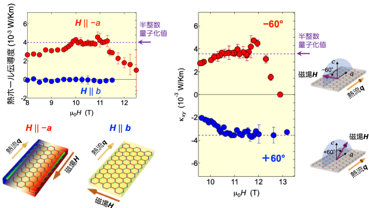
図1：（左上）面内磁場( H \parallel -a , H \parallel b )における \alpha -RuCl 3 の熱ホール伝導度の磁場依存性。 H \parallel -a において、磁場を変化させると、ある磁場範囲で熱ホール伝導度が量子化熱伝導度の1/2で一定となり、半整数熱量子ホール効果が観測された。一方、 H \parallel b では熱ホール伝導度はほぼゼロとなった。（左下） H \parallel -a , H \parallel b における熱ホール効果のイメージ図。（右）傾斜磁場( \pm 60^\circ )における熱ホール伝導度の磁場依存性。 +60^\circ と -60^\circ で半整数熱量子ホール効果の符号が反転する。
